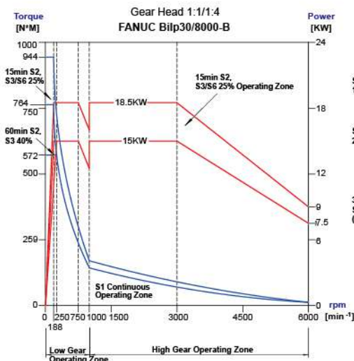
BT50 Gear head 6000rpm
