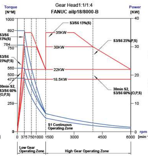
BT50 Gear head 6000rpm
